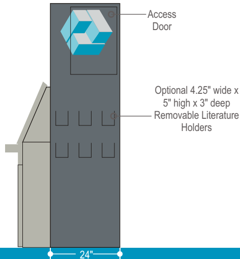
MINI KIOSK RIGHT ELEVATION (DEPARTURE)
